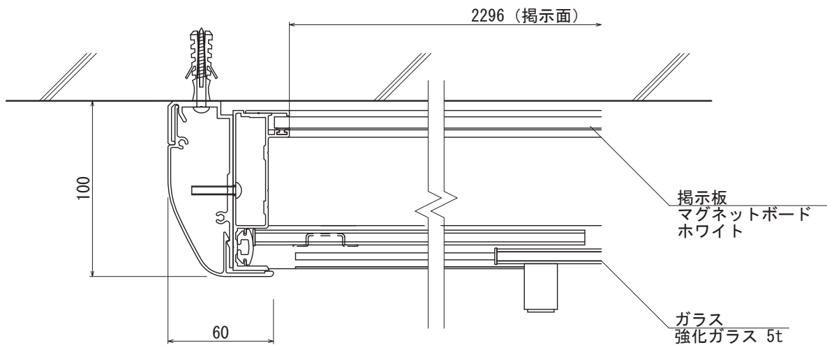
【平面図 S=1:3】
