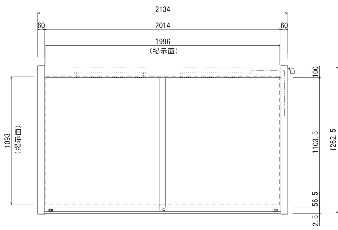
【正面図 S=1:20】
