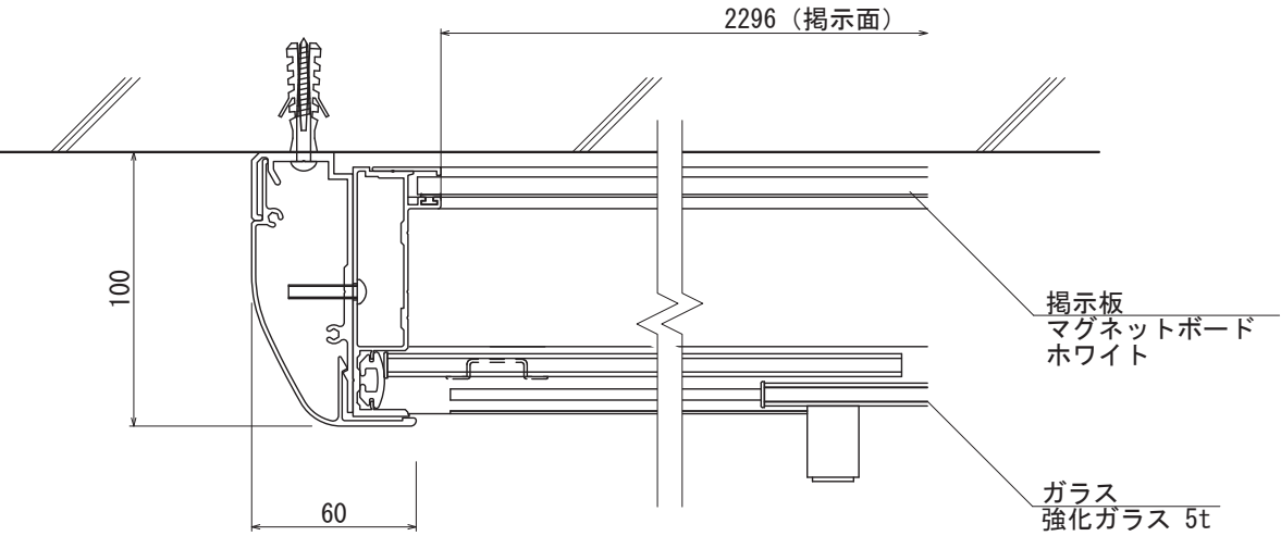
【平面図 S=1:3】
