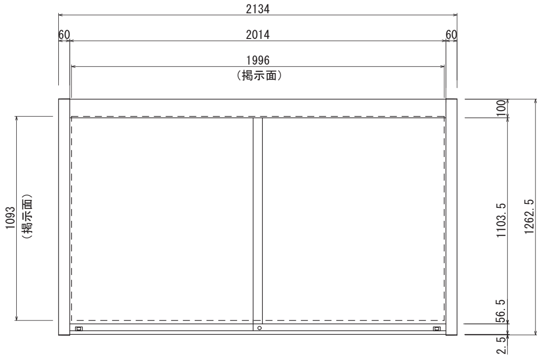
【正面図 S=1:20】
