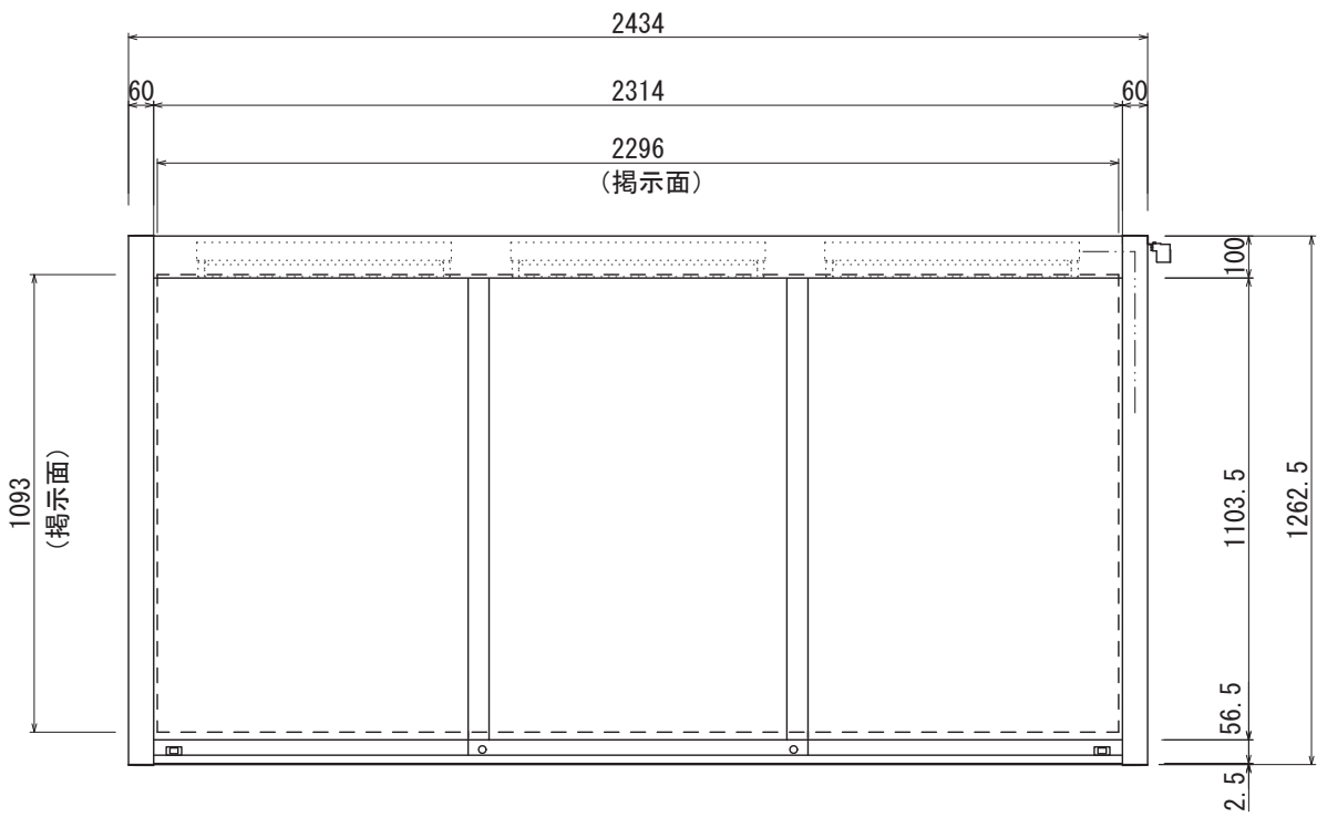
【正面図 S=1:20】
