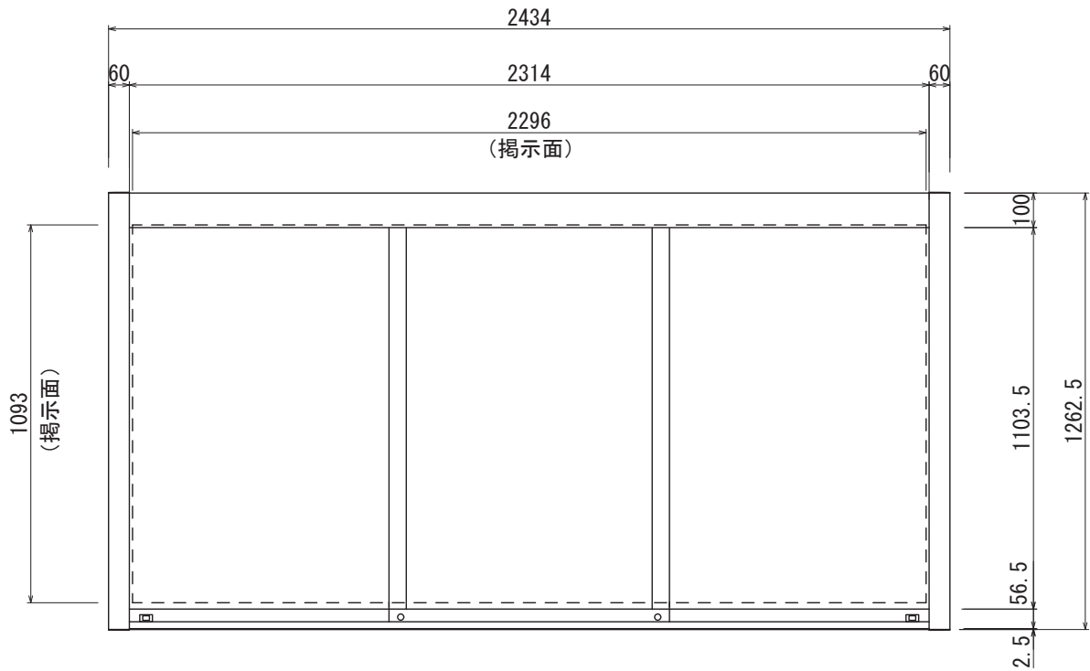
【正面図 S=1:20】
