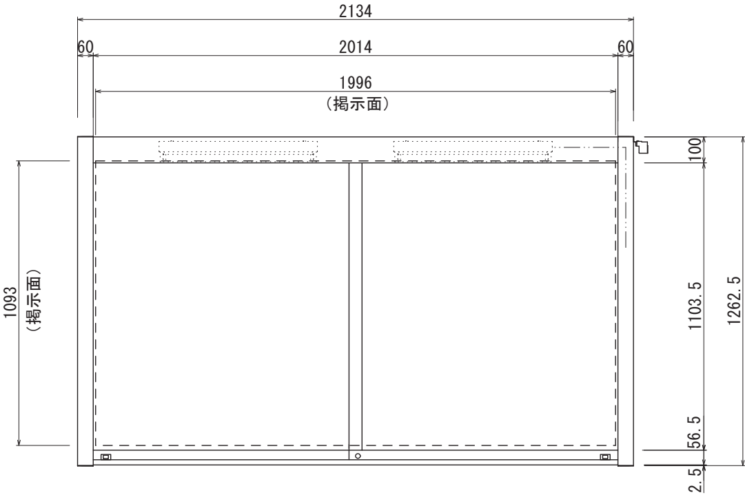
【正面図 S=1:20】
