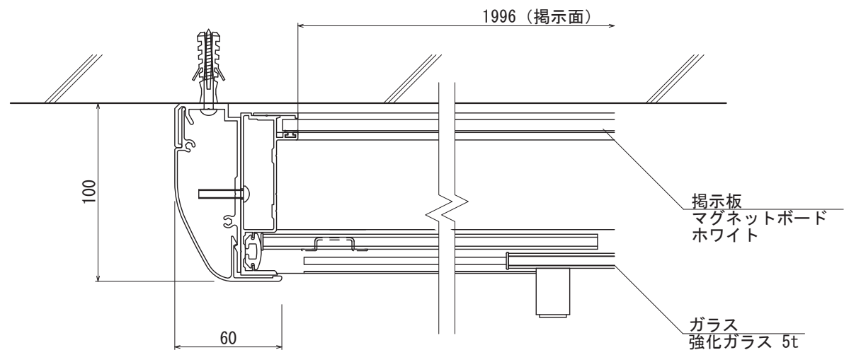
【平面図 S=1:3】
