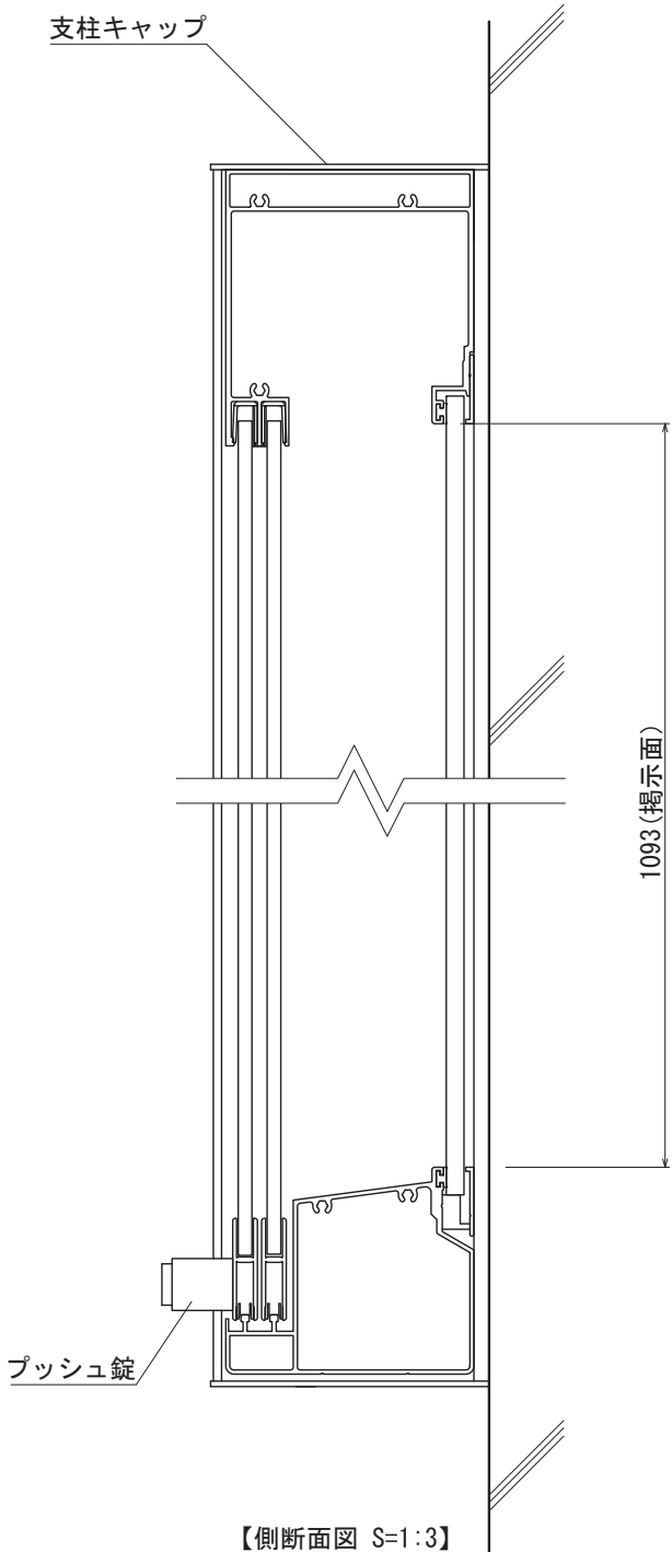
【側断面図 S=1:3】
