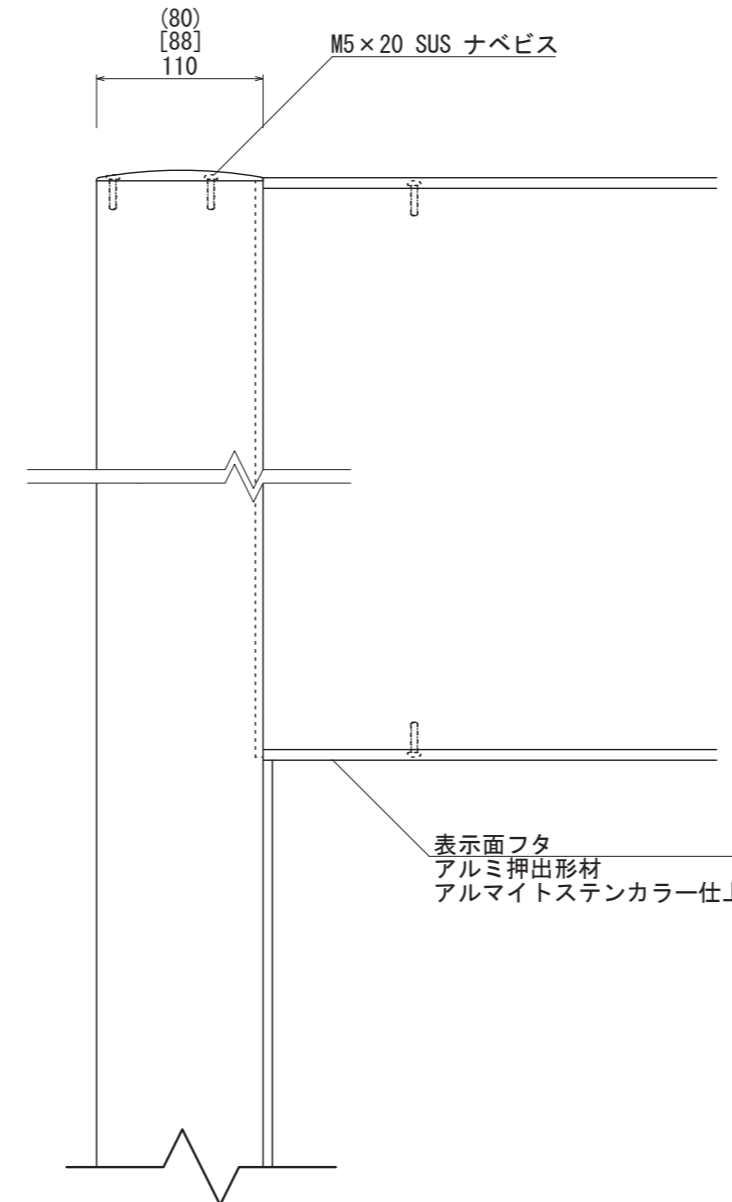
【正面図 S=1:5】
