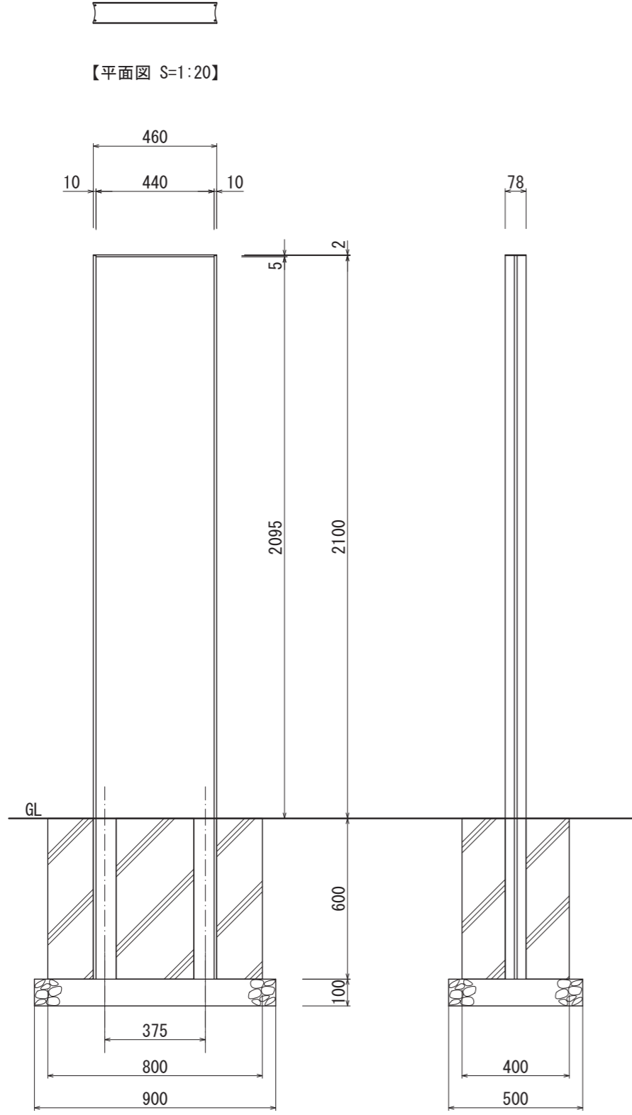
【正面図 S=1:20】
