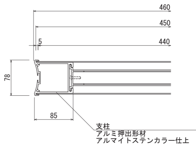
【平面図 S=1:5】
