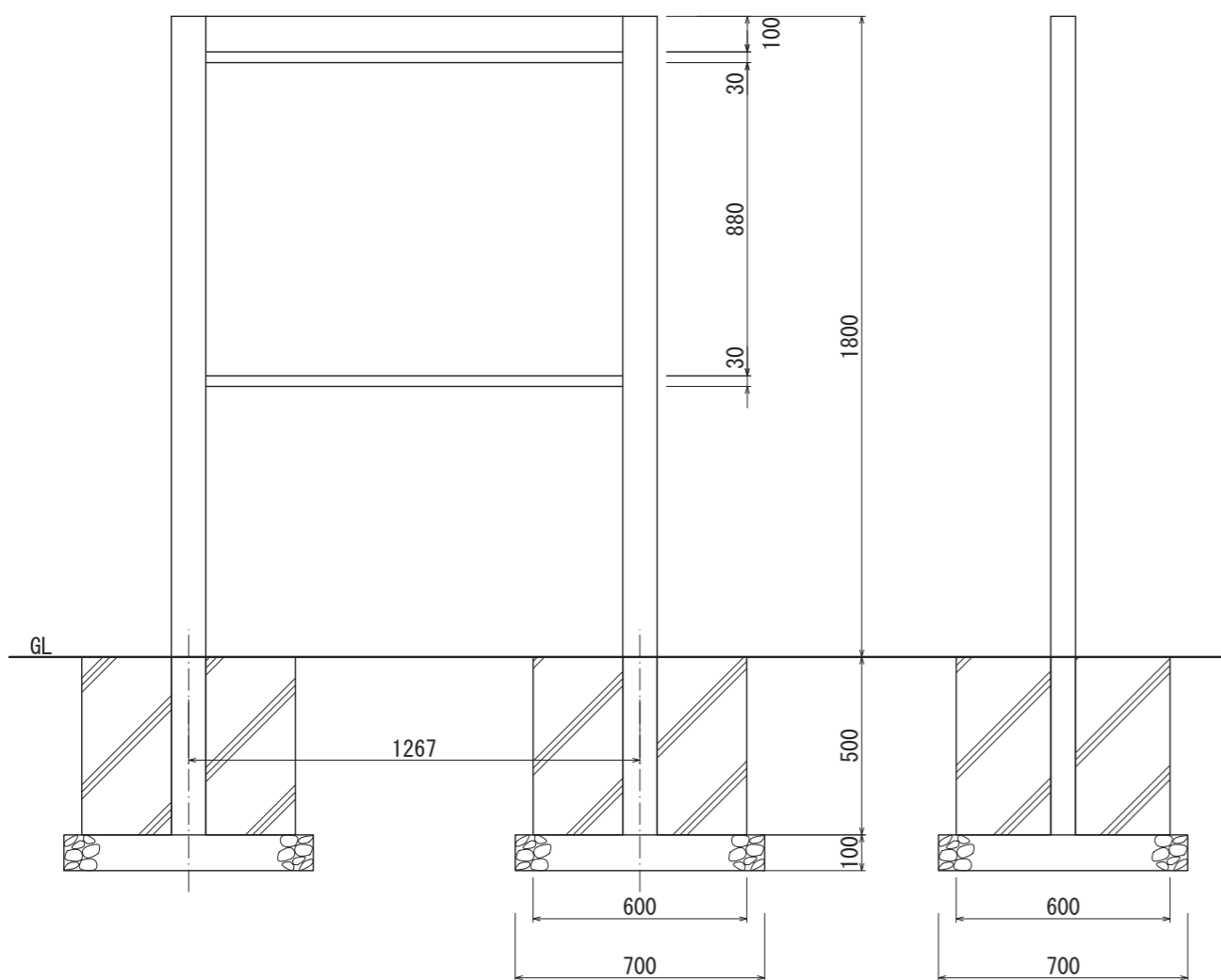
【正面図 S=1:20】
