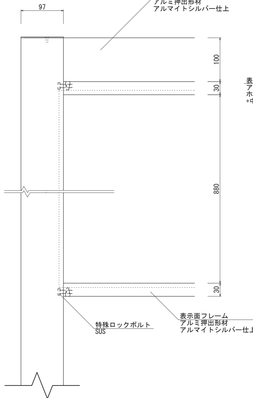
【正面図 S=1:5】
