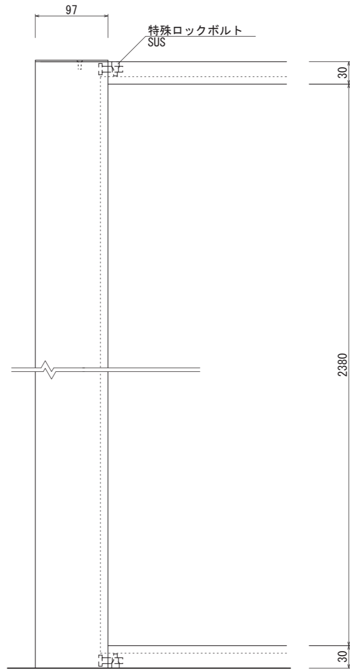
【正面図 S=1:5】
