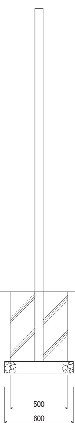
【側面図 S=1/20】
