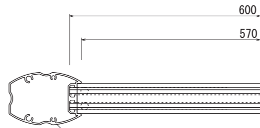
【平面図 S=1:5】
