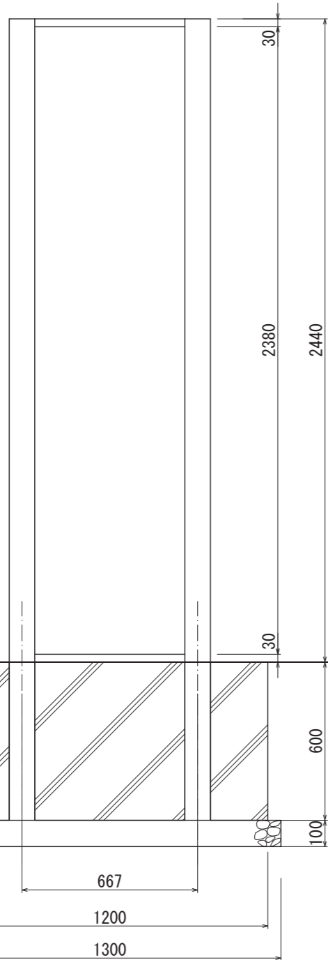
【正面図 S=1/20】
