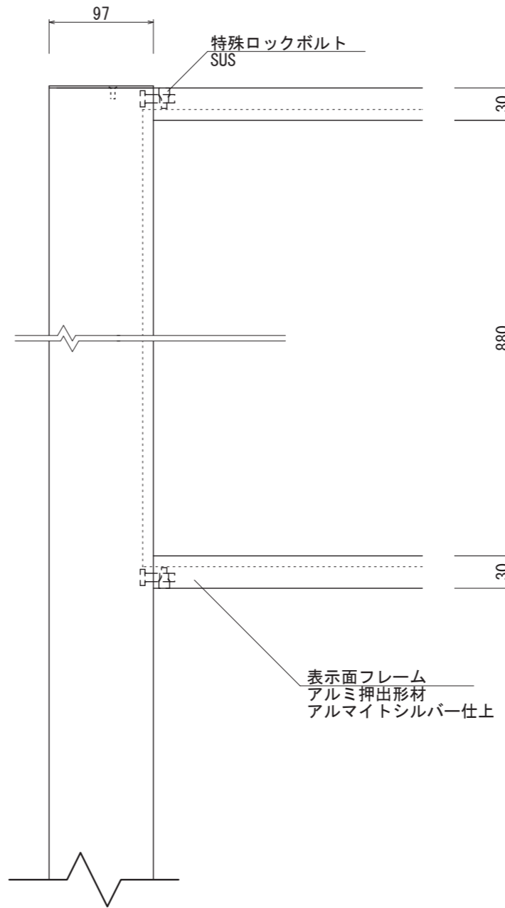
【正面図 S=1:5】
