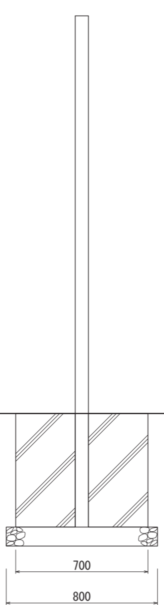
【側面図 S=1:20】
