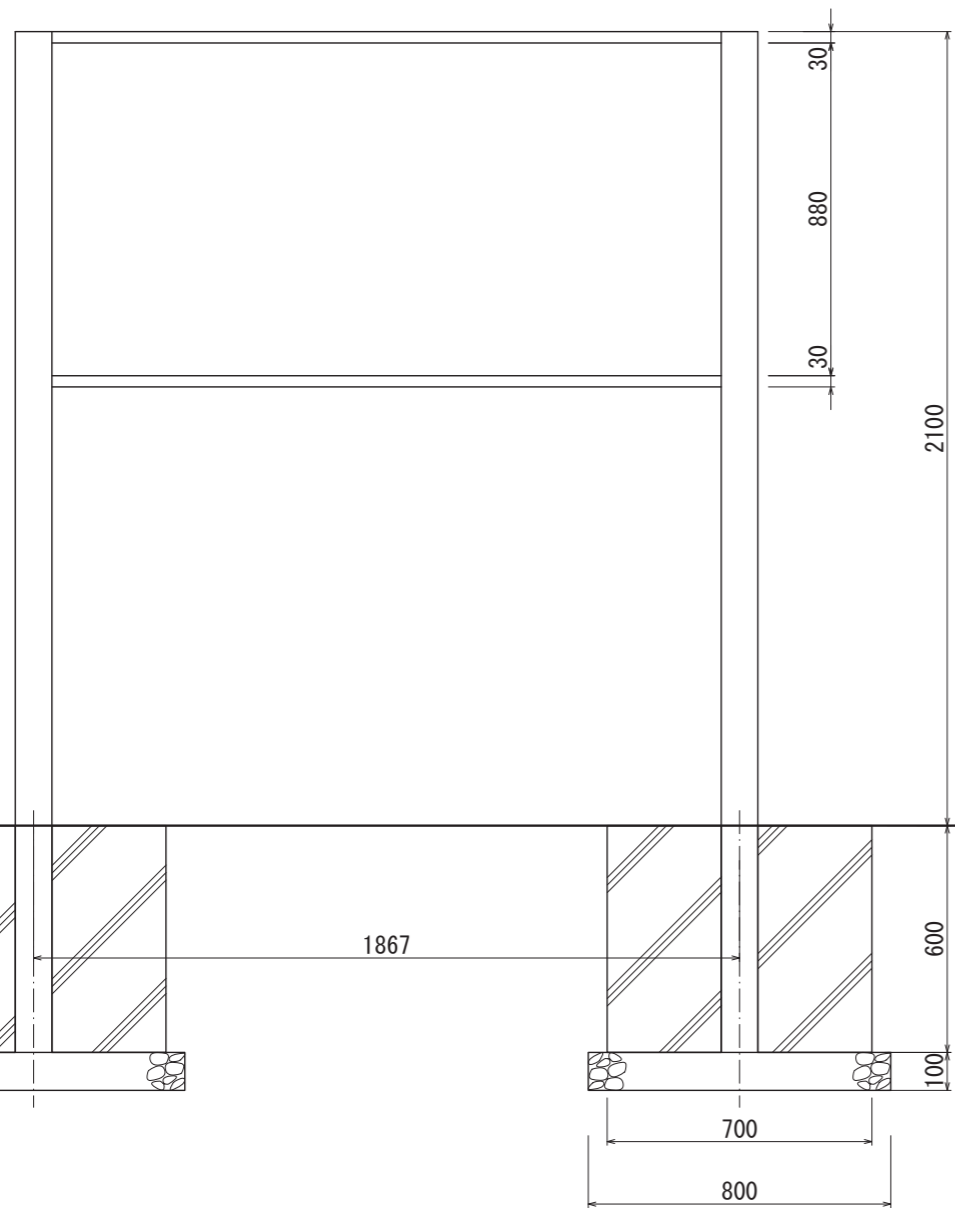
【正面図 S=1:20】
