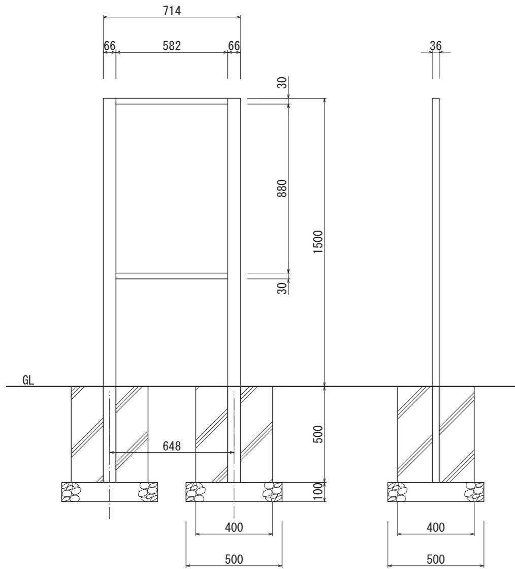
【正面図 S=1:20】
