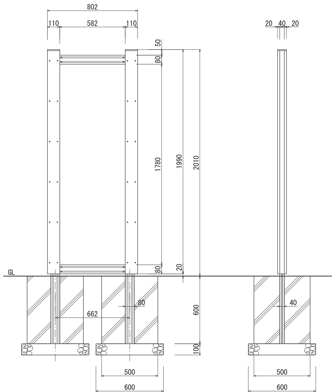
【正面図 S=1:20】
