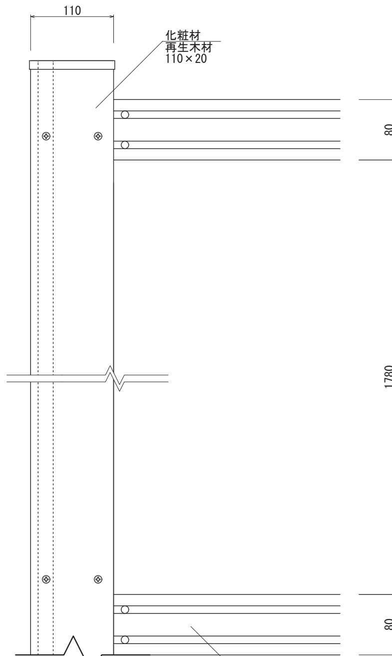
【正面図 S=1:5】
