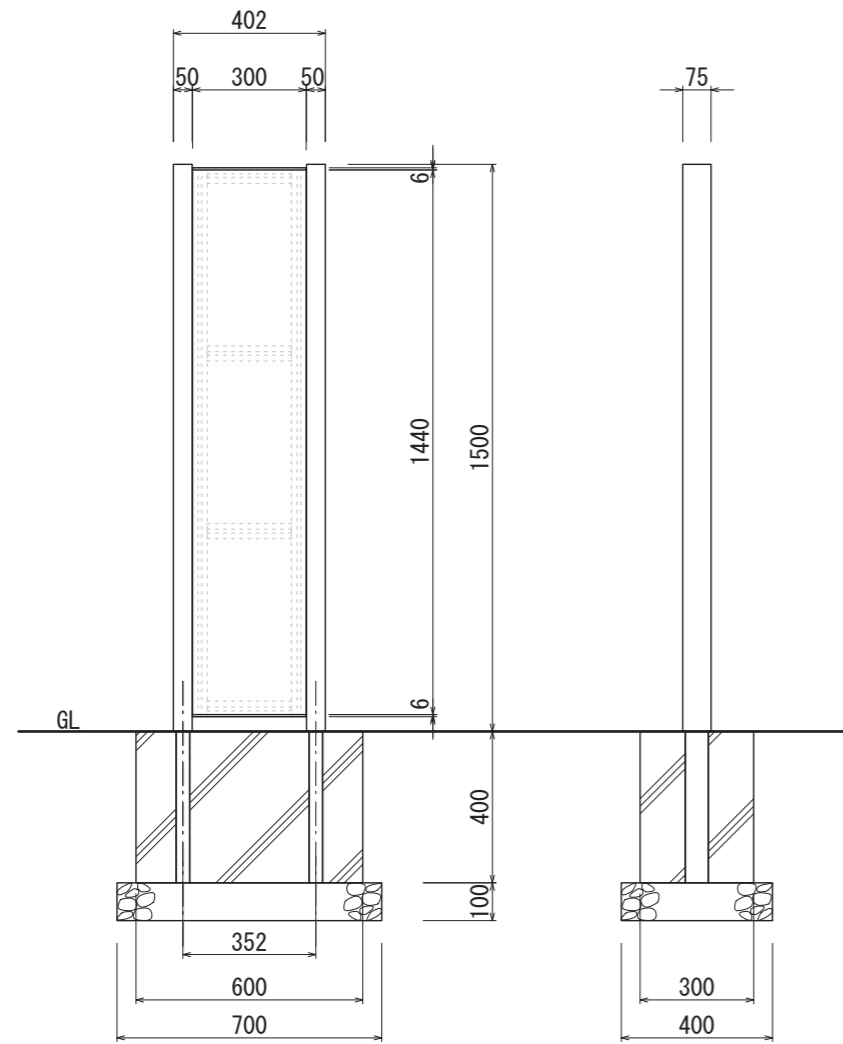
【正面図 S=1:20】
