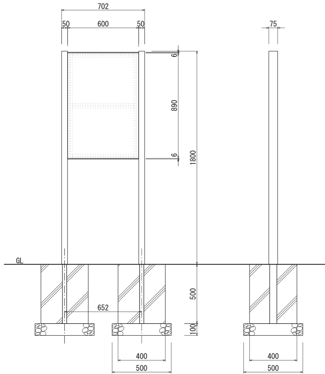
【正面図 S=1:20】
