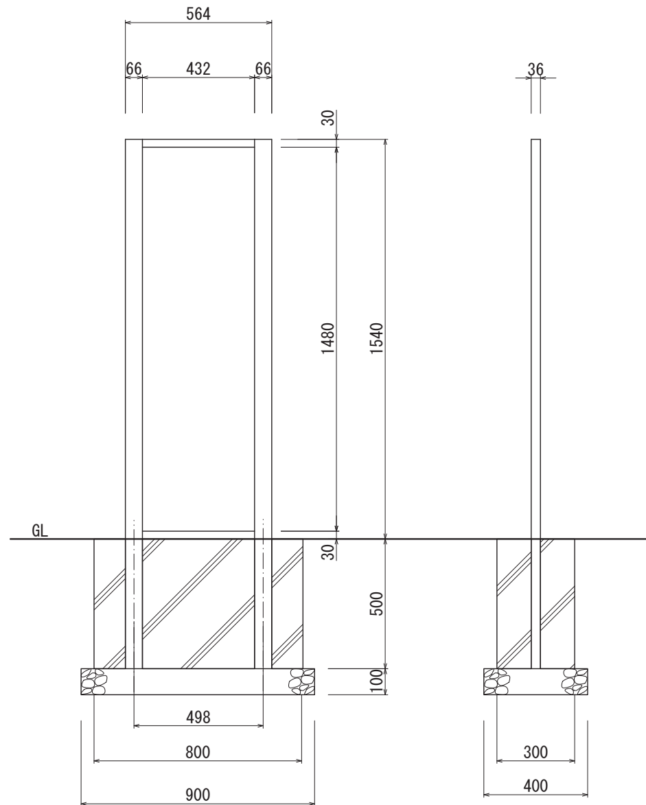
【正面図 S=1:20】
