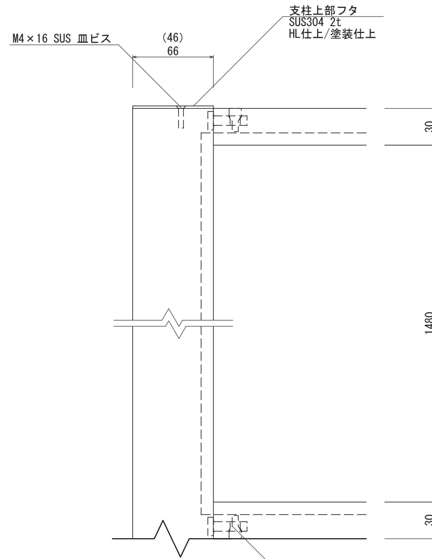
【正面図 S=1:3】
