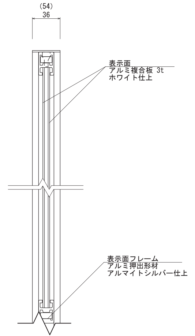
【断面図 S=1:3】
