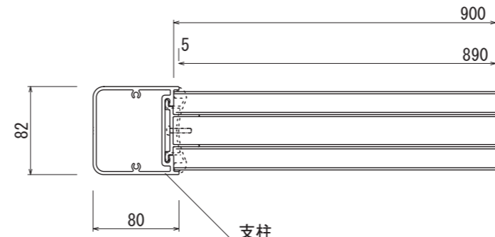
【平面図 S=1:5】
