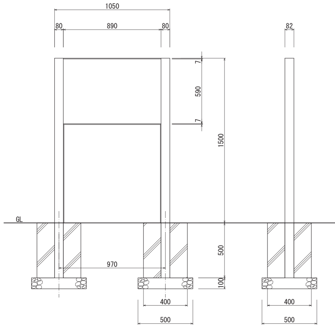
【正面図 S=1:20】
