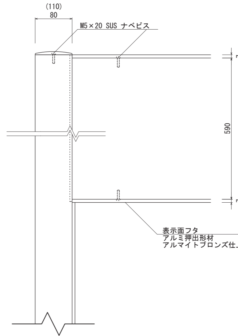
【正面図 S=1:5】
