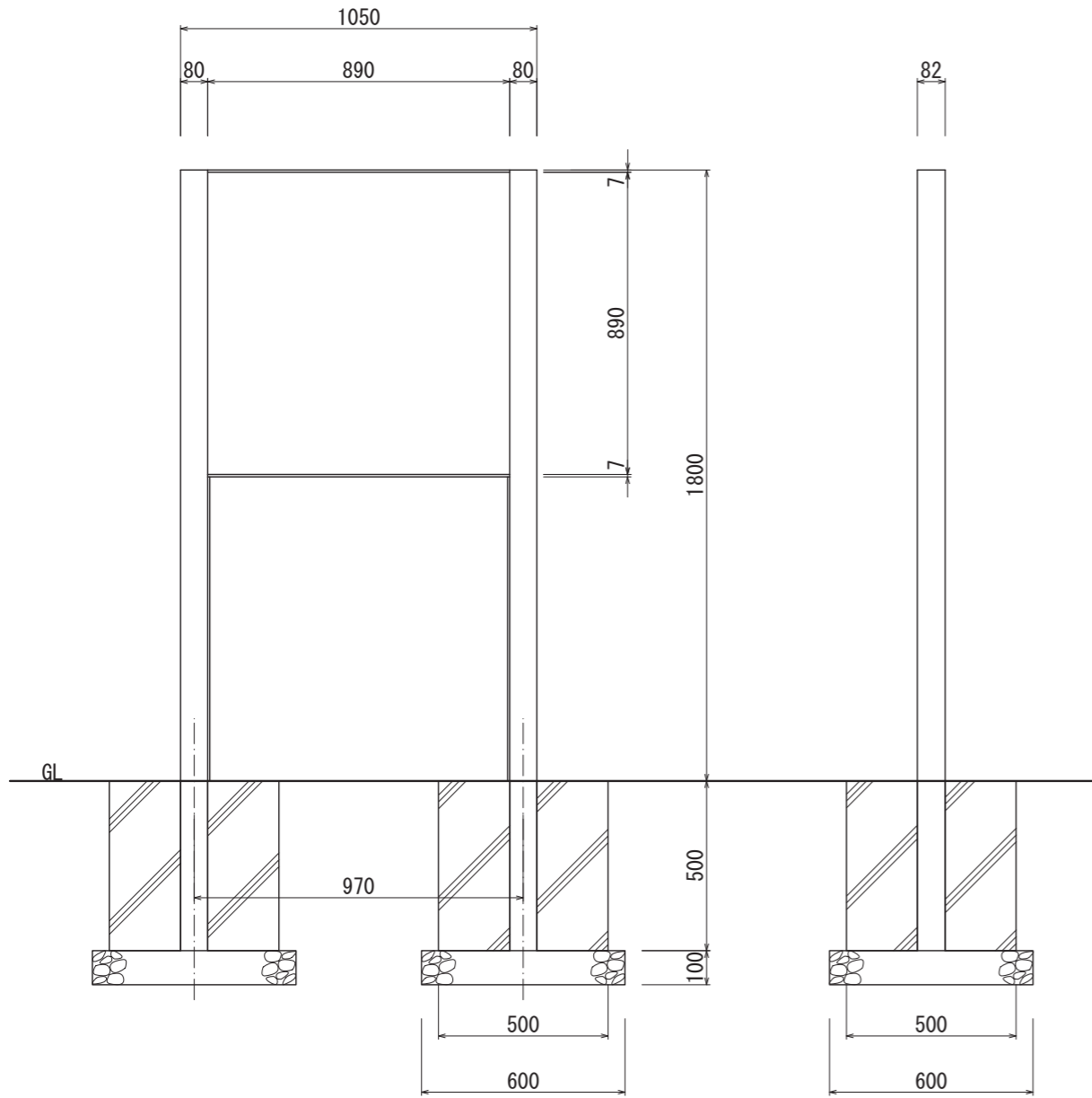
【正面図 S=1:20】
