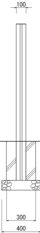
【側面図 S=1:20】
