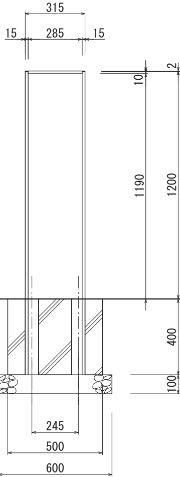
【正面図 S=1:20】
