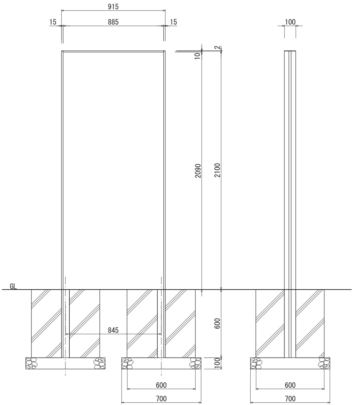
【正面図 S=1:20】
