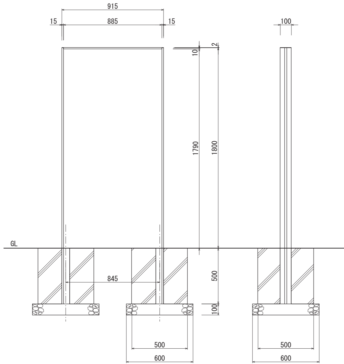
【正面図 S=1:20】
