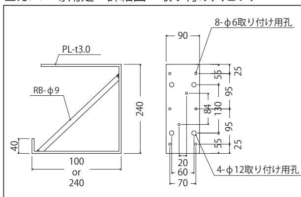
■カバー専用足 詳細図 取り付け穴ピッチ
