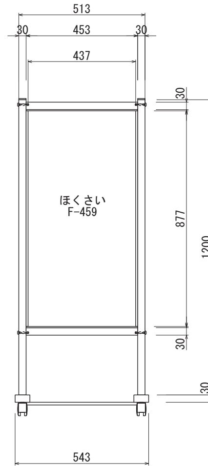
【正面図 S=1:15】
