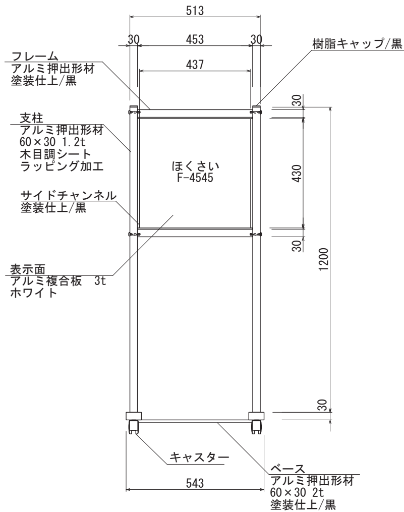
【正面図 S=1:15】
